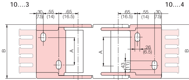
1015-34P(Z) - 1050-34P(Z)
