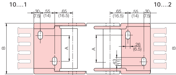
1015-12P(Z) - 1050-12P(Z)
